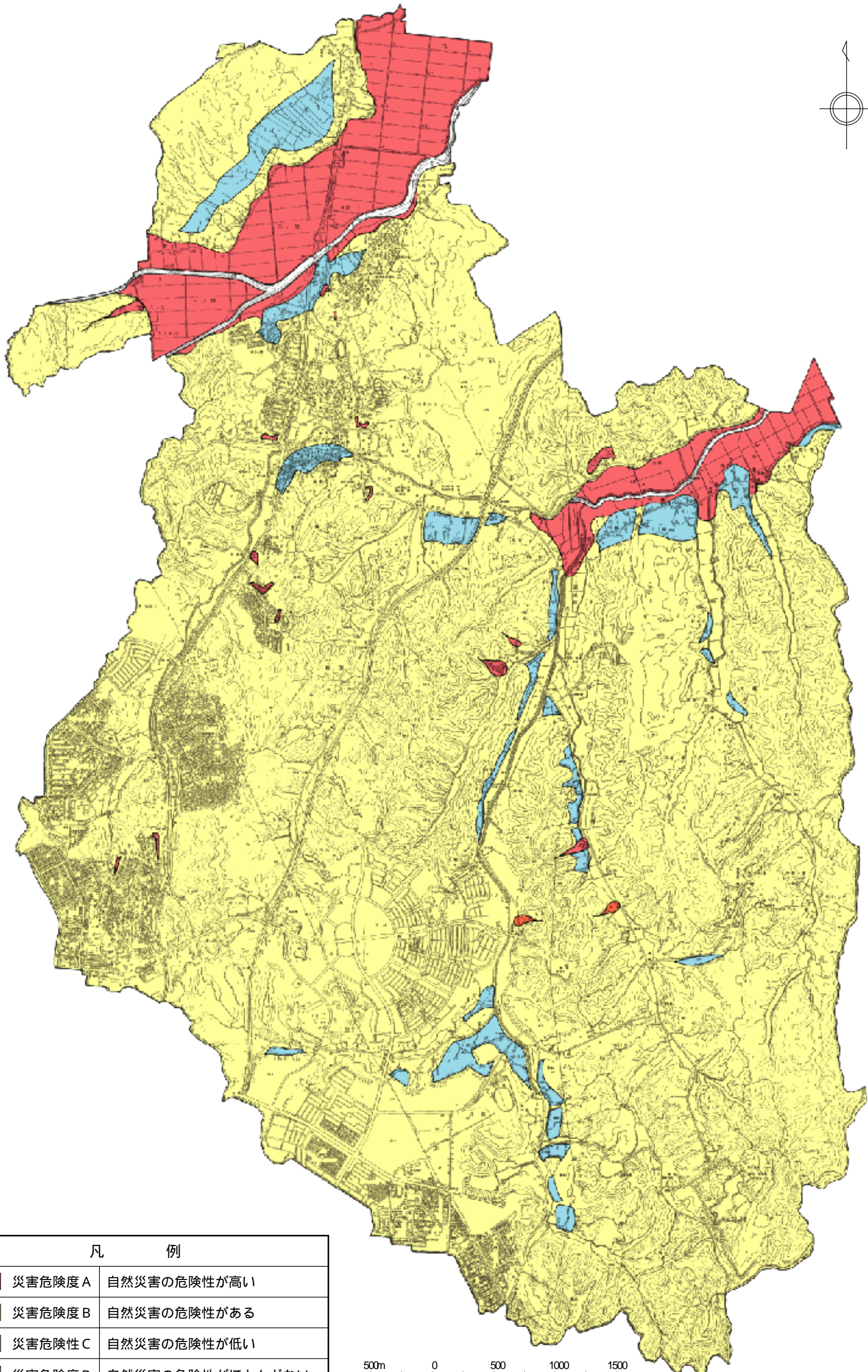
災害総合評価図
